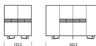
MADIA CREDENZA L 123.2-L 243.2 P 48.8 H 153 CRÉDENCE
