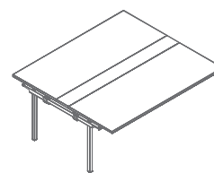
SY18 1800 / 1610 / 740 80.3 kg
